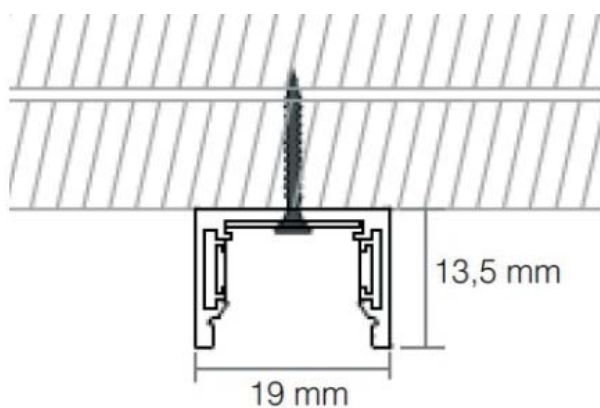
Unión angular 90° empotrado y superficie
